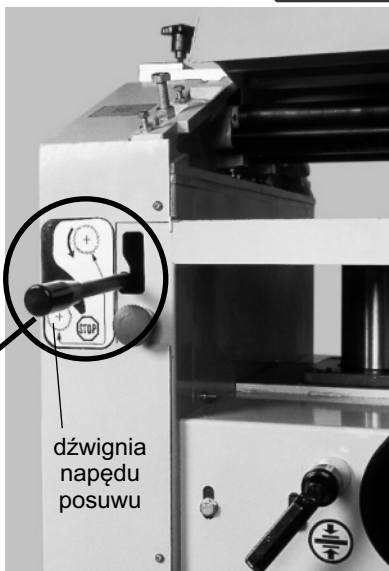
C) Piktogram przełączenia dźwigni napędu posuwu
